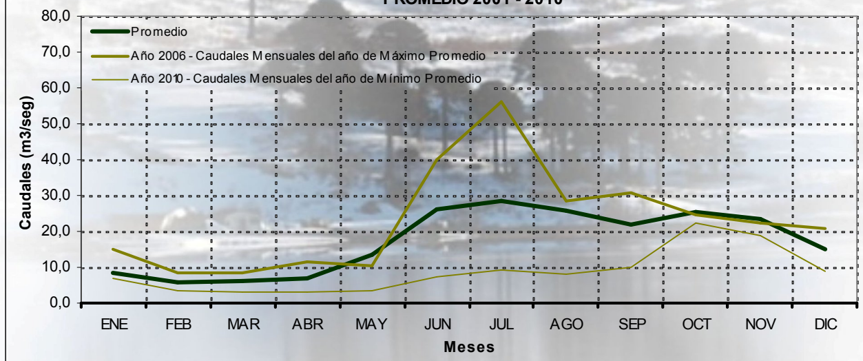
CAUDAL PROMEDIO - CAUDALES MENSUALES DEL AÑO DE MÁXIMO Y MÍNIMO PROMEDIO 2001 - 2010
